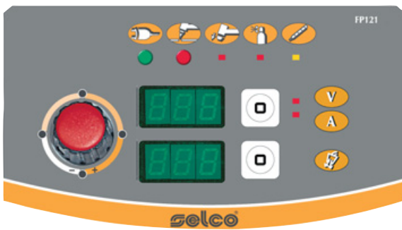
Panneau de commandes du modèle Genesis 60 Panel de mandos de Genesis 60 Bedieningspaneel van de Genesis 60
